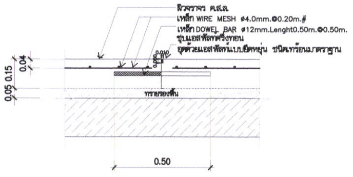
แบบขยาย LONGTUDNAL JOINT
