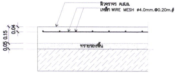
แบบขยาย C (ขยายรูปตัดแนวริม)
